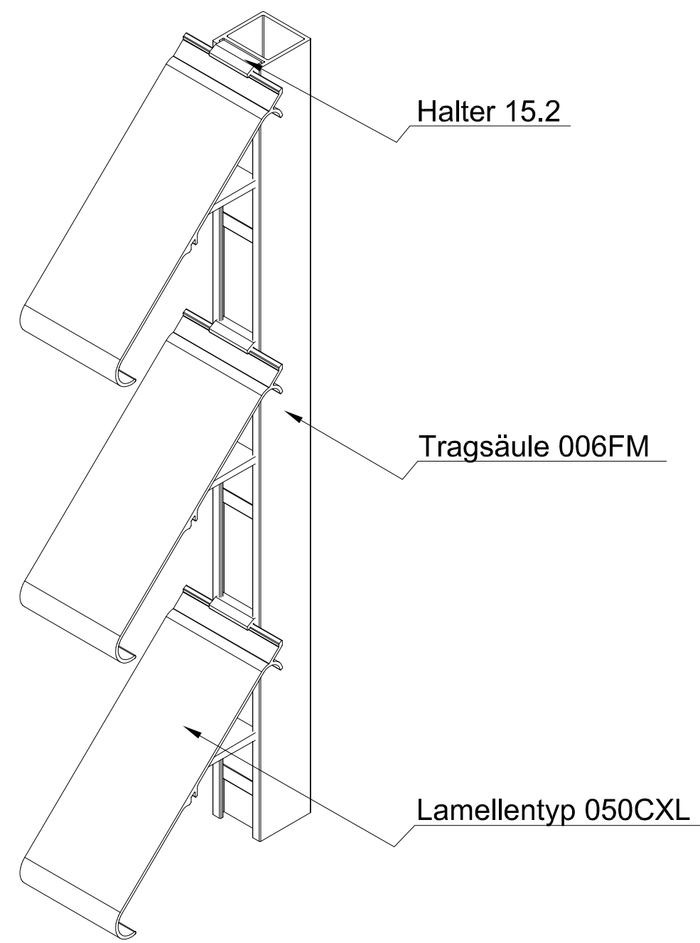
ISO-Ansicht
