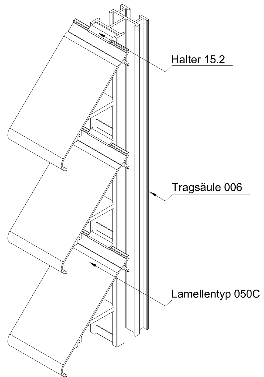
ISO-Ansicht
