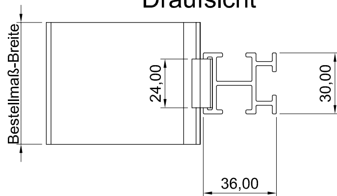
Draufsicht
