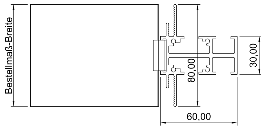
Draufsicht
