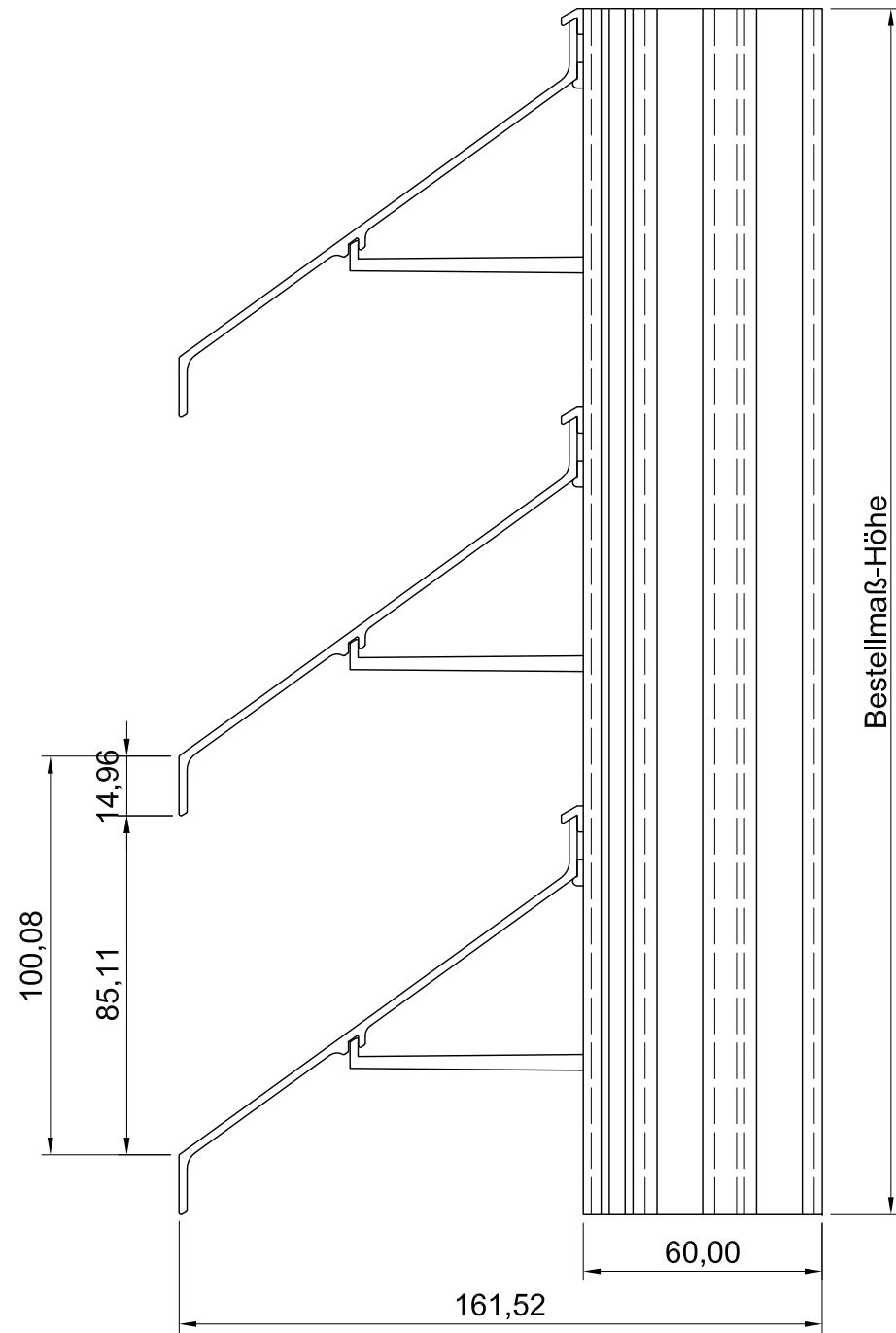
Draufsicht
