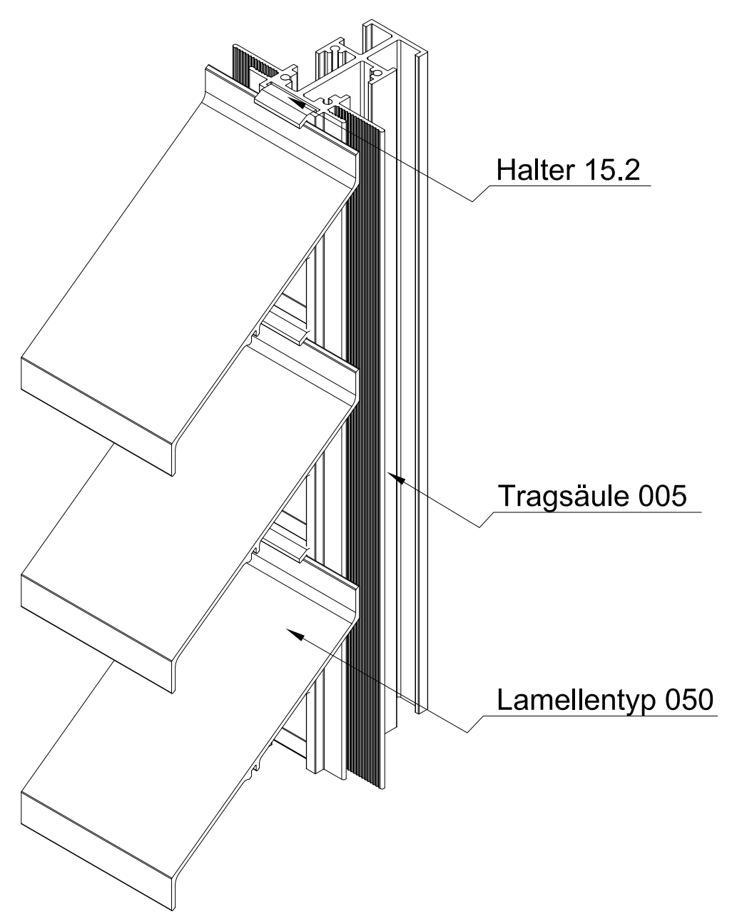
ISO-Ansicht
