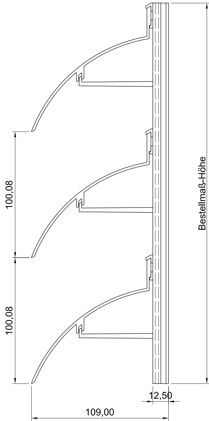
Seitenansicht
