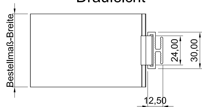
Draufsicht
