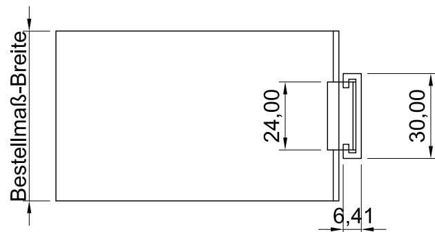
Draufsicht
