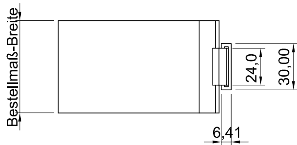
Draufsicht
