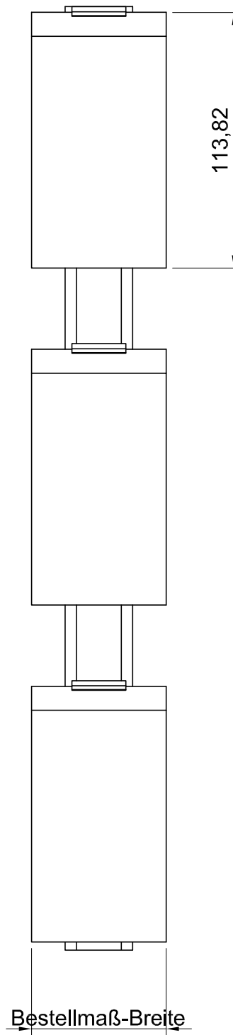
Seitenansicht
