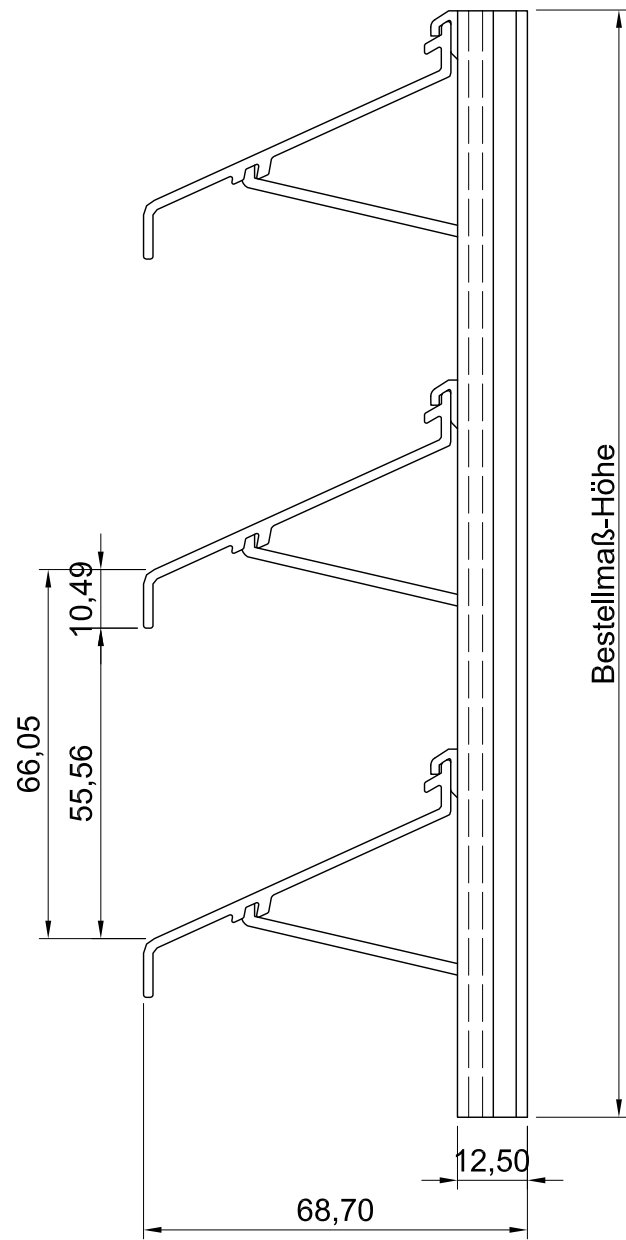
Seitenansicht
