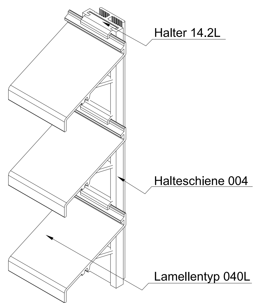
ISO-Ansicht
