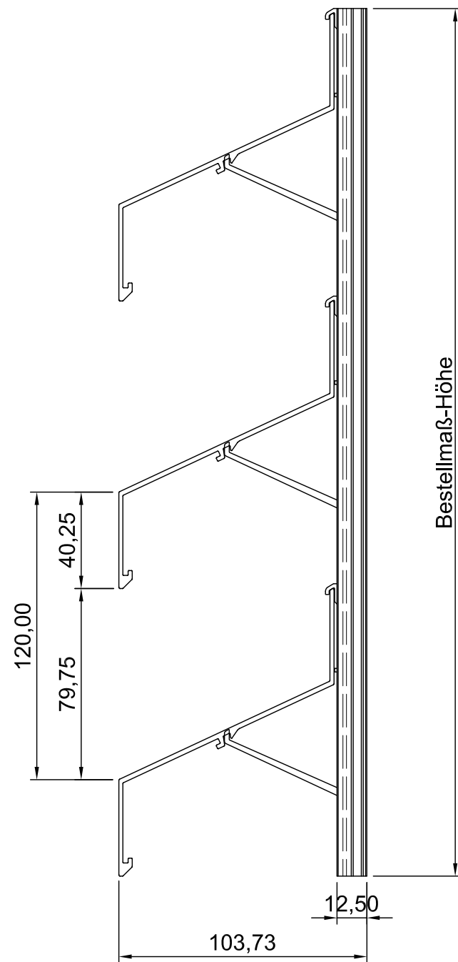
Seitenansicht
