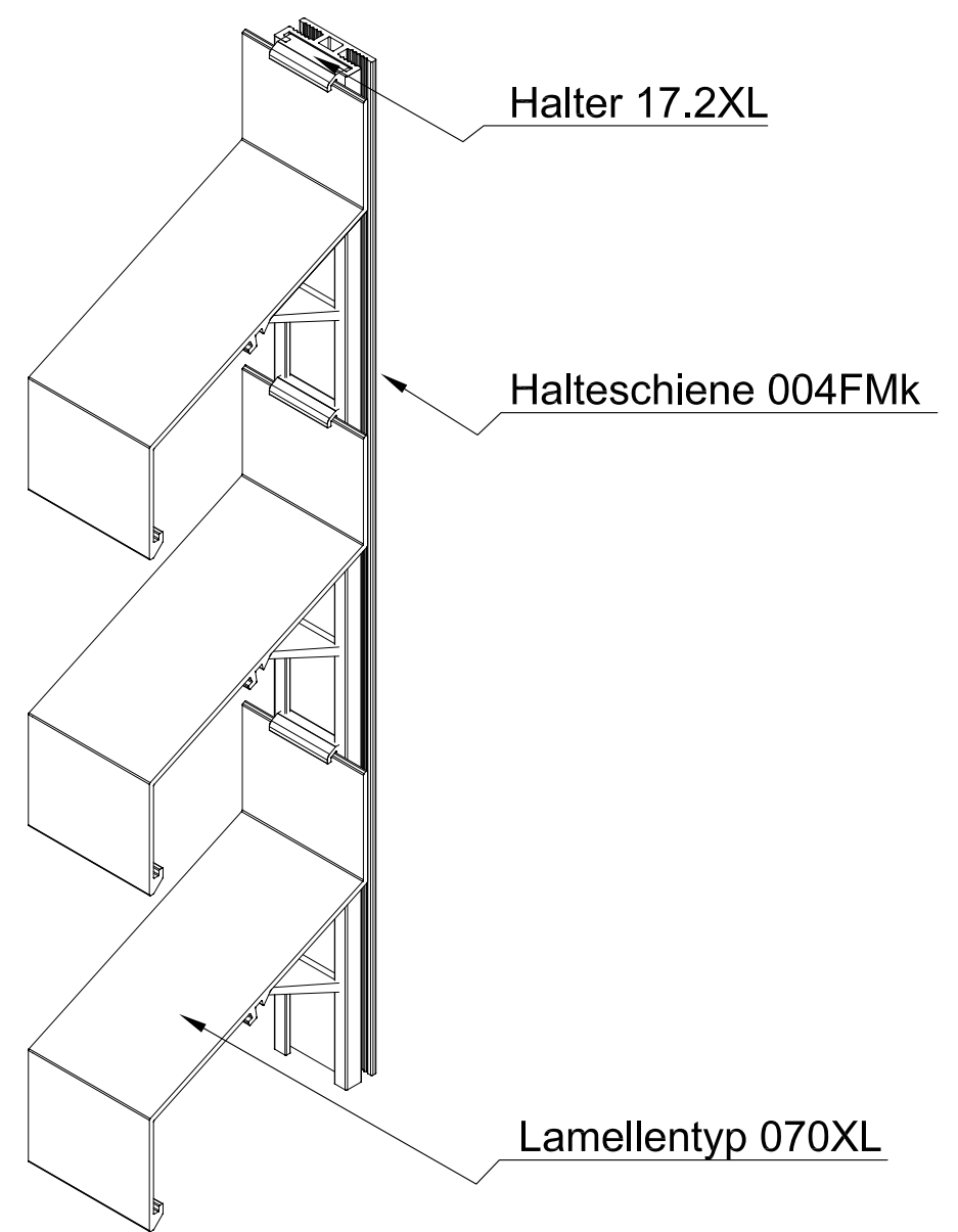
ISO-Ansicht
