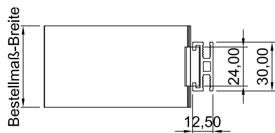
Draufsicht
