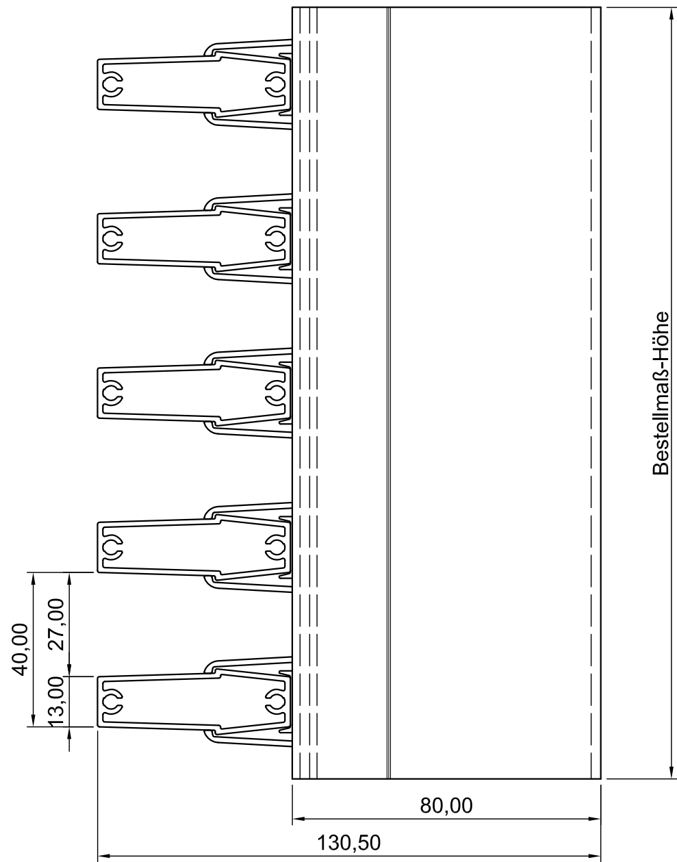
Seitenansicht
