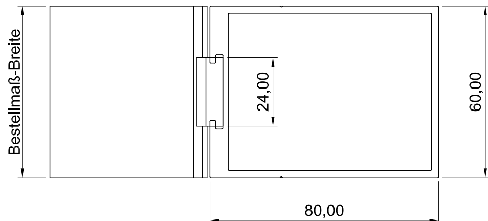
Draufsicht
