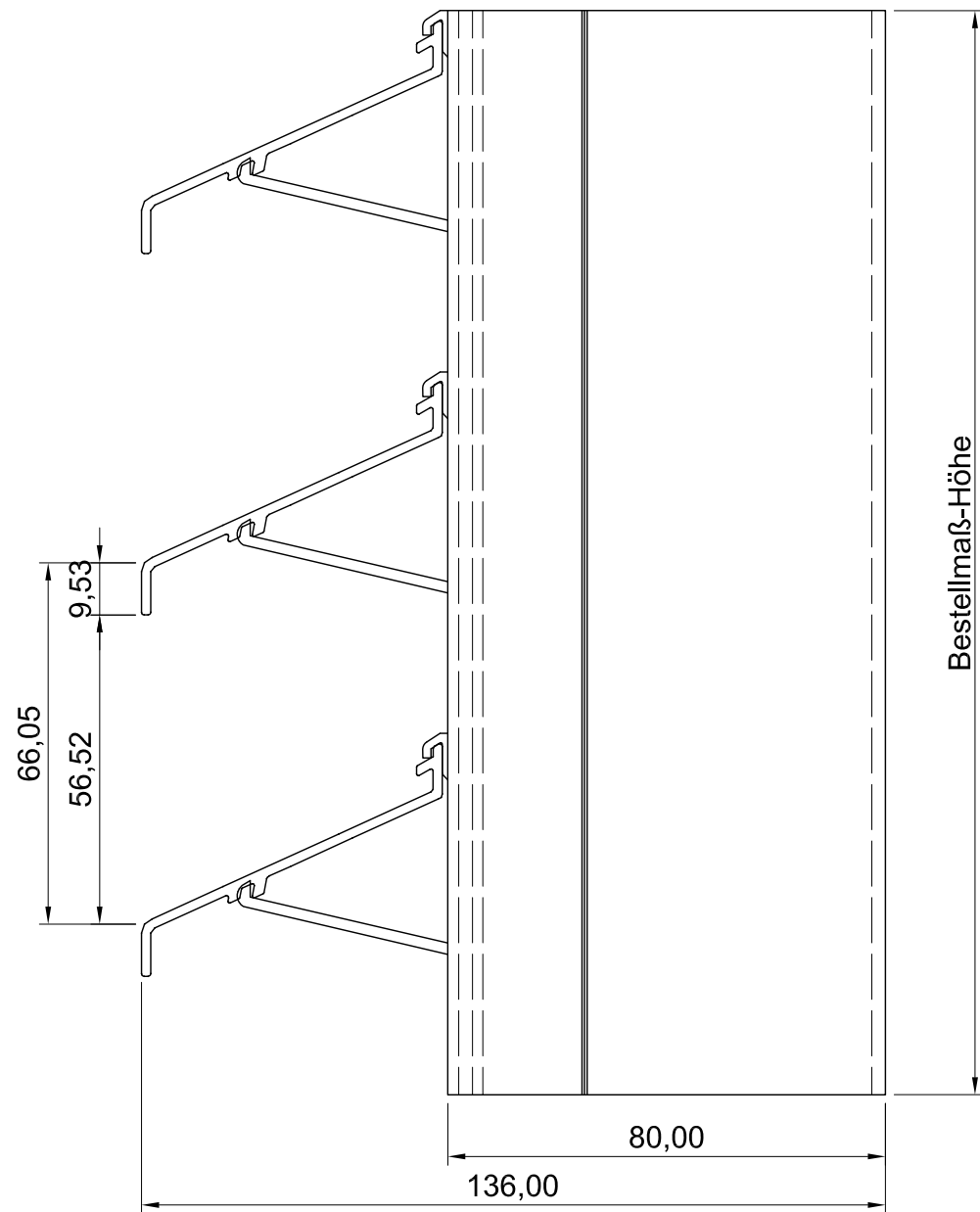
Seitenansicht
