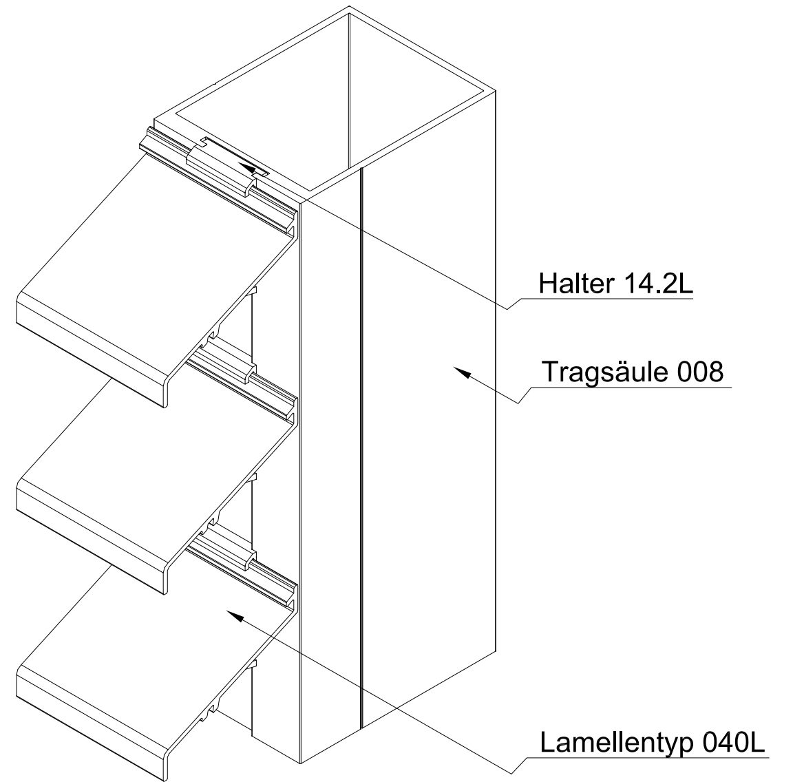
ISO-Ansicht
