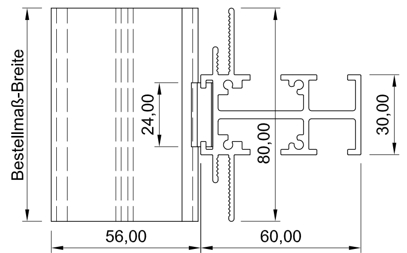
Draufsicht
