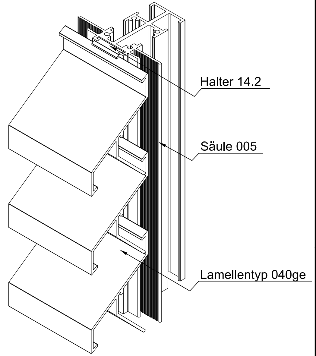
ISO-Ansicht
