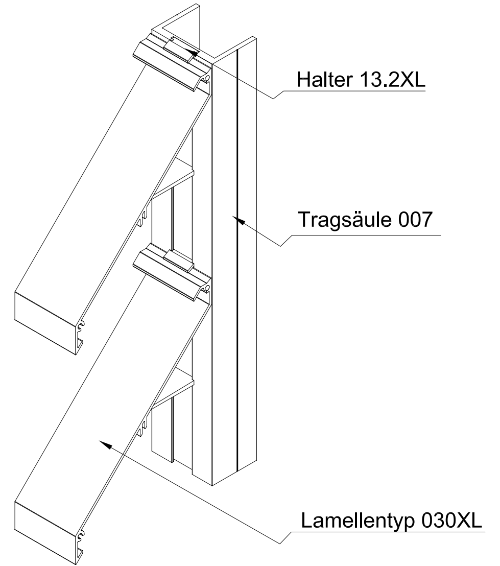
ISO-Ansicht
