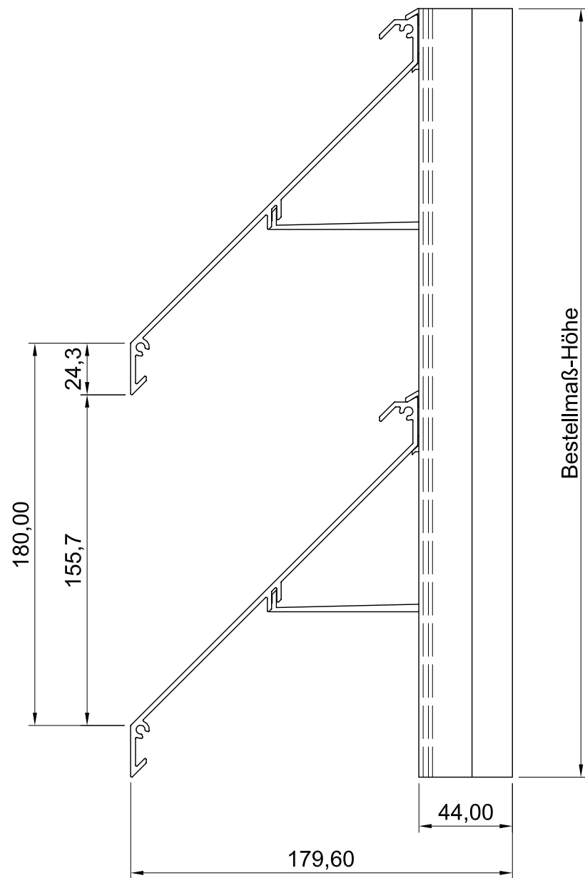
Seitenansicht
