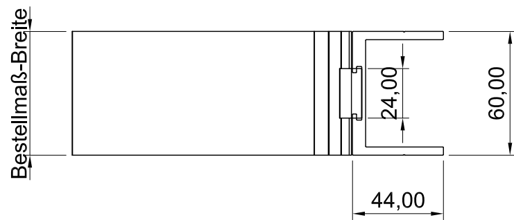
Draufsicht
