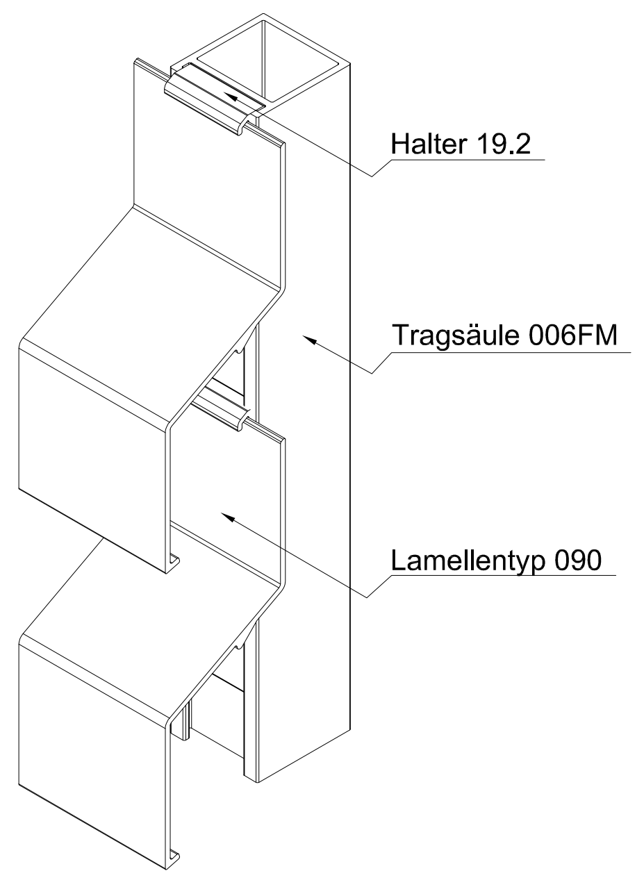
ISO-Ansicht
