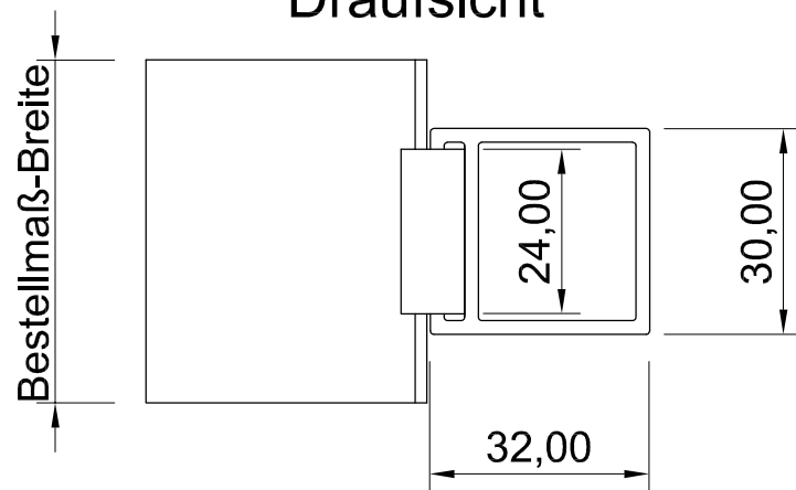
Draufsicht
