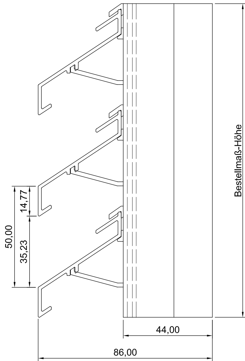
Seitenansicht
