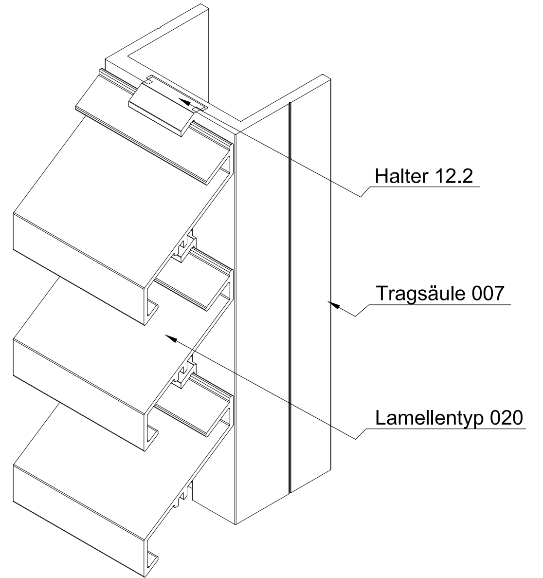
ISO-Ansicht
