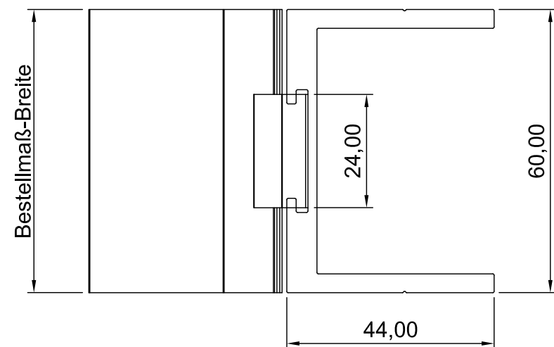
Draufsicht
