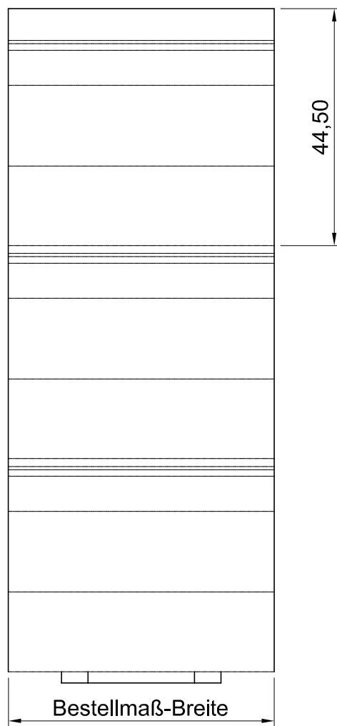
Vorderansicht
