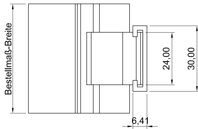
Draufsicht
