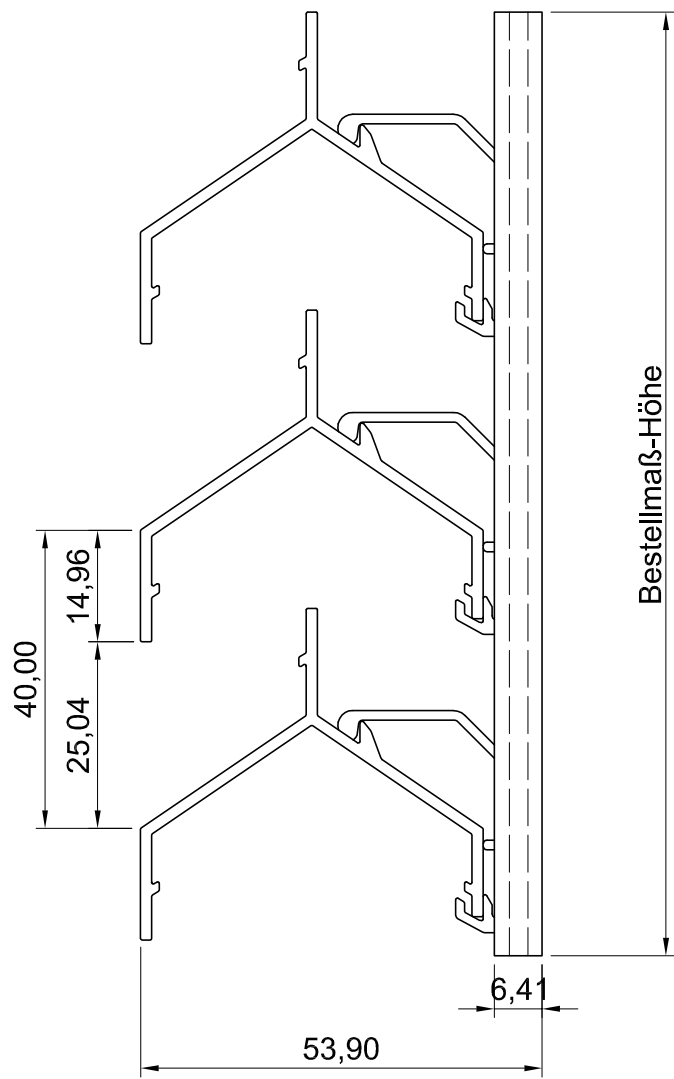
Seitenansicht
