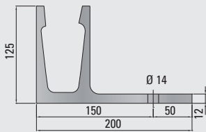
Bohrbild (Ø 14 mm)
